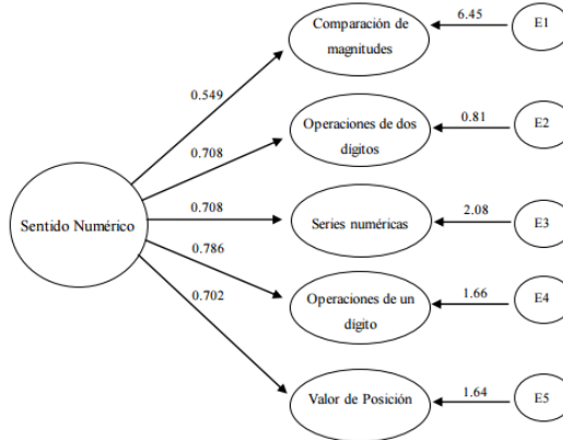
Figura 3. Modelo de un factor general. IPAM Forma C
