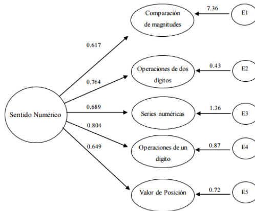
Figura 1. Modelo de un factor general. IPAM Forma A
