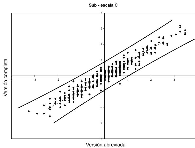
Figura 3 Comparación de las medidas obtenidas con la versión abreviada y la completa, subescala C
